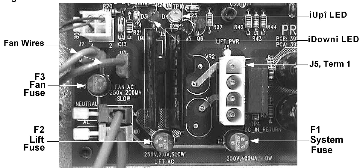
Diagram 5.2 ó Lower PCA
